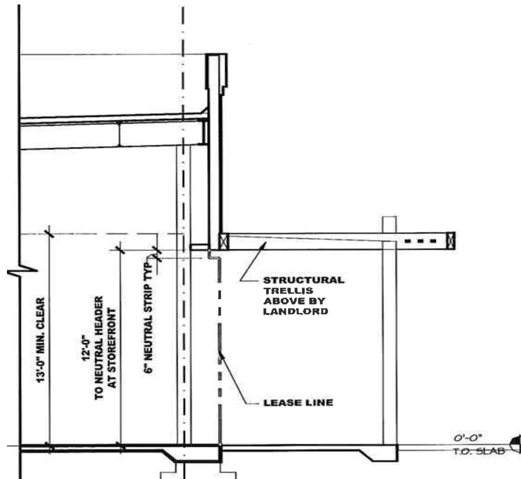
TENANT STOREFRONT ZONES - ZONE 7 - LEVEL TWO SECTION
