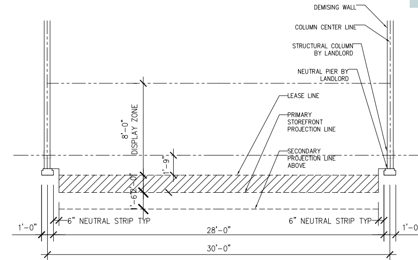
TENANT STOREFRONT ZONES - ZONE 3 - LEVEL ONE PLAN
