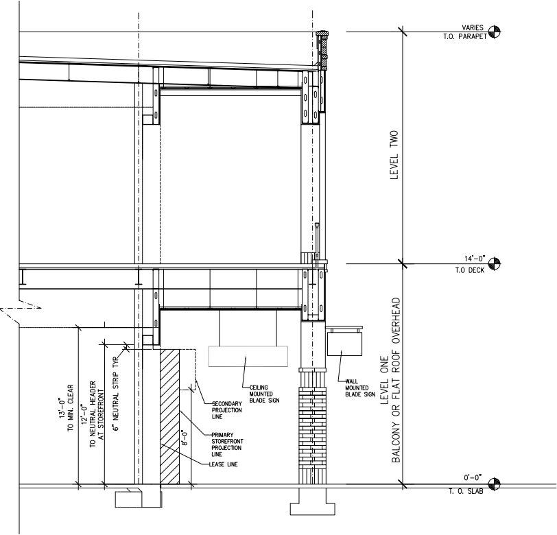
TENANT STOREFRONT ZONES - ZONE 1 - LEVEL ONE SECTION
