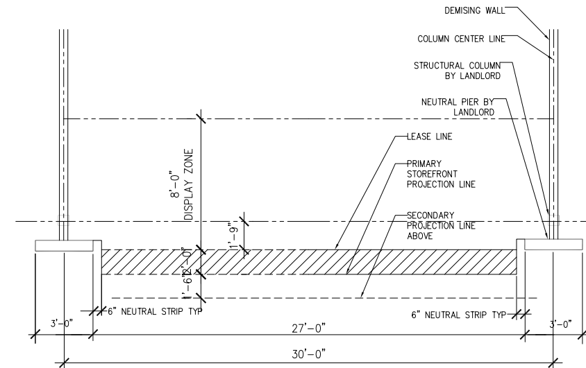
TENANT STOREFRONT ZONES - ZONE 4 - LEVEL TWO PLAN
