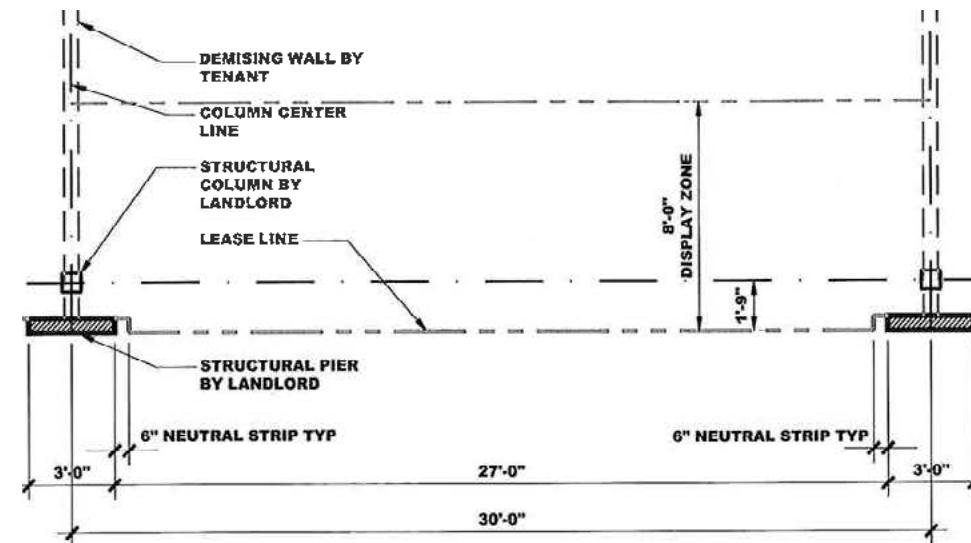
TENANT STOREFRONT ZONES - ZONE 7 - LEVEL TWO PLAN
