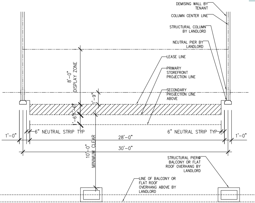
TENANT STOREFRONT ZONES - ZONE 1 - LEVEL ONE PLAN
