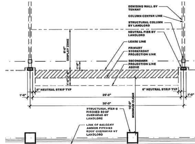
TENANT STOREFRONT ZONES - ZONE 5 - LEVEL TWO PLAN
