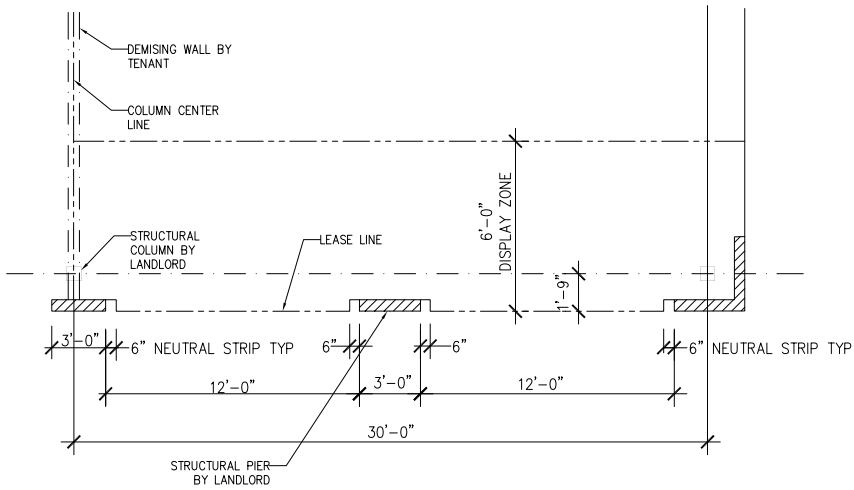
TENANT STOREFRONT ZONES - ZONE 2 - LEVEL ONE PLAN
