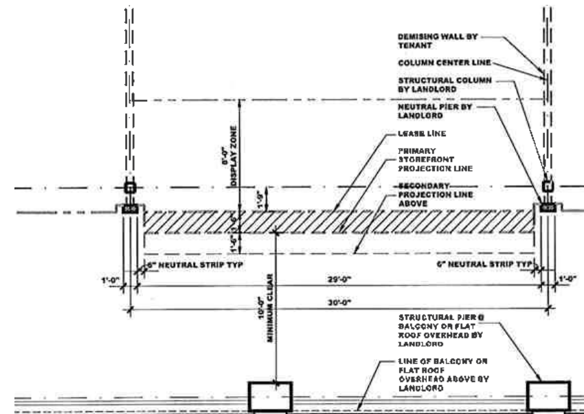
TENANT STOREFRONT ZONES - ZONE 6 - LEVEL TWO PLAN
