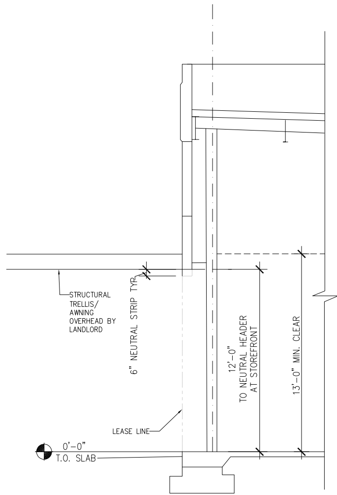
TENANT STOREFRONT ZONES - ZONE 2 - LEVEL ONE SECTION
