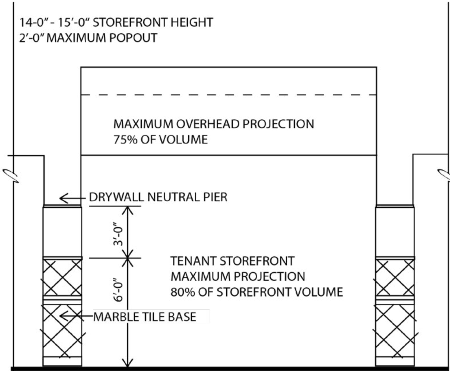
ELEVATION
