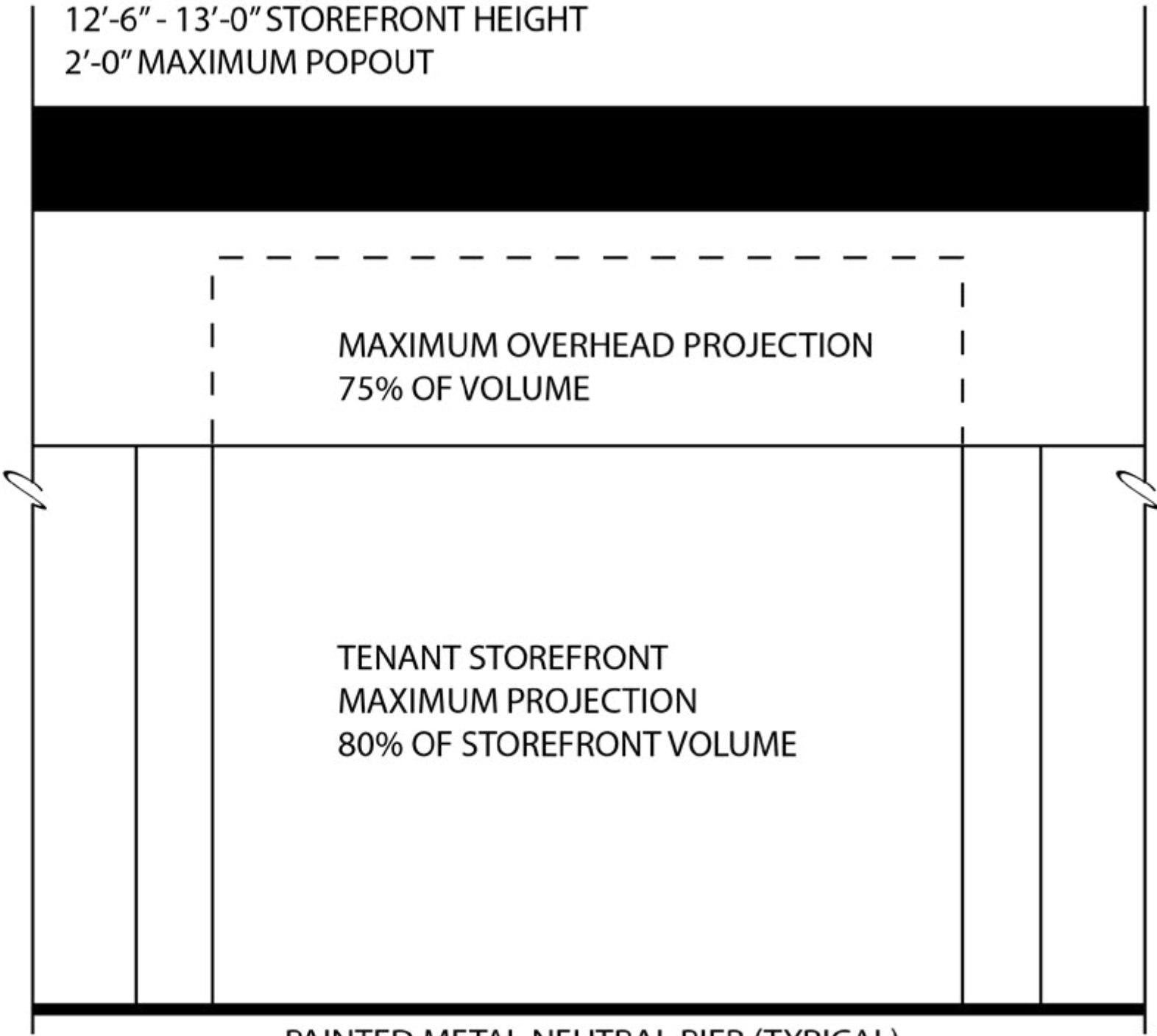
ELEVATION
