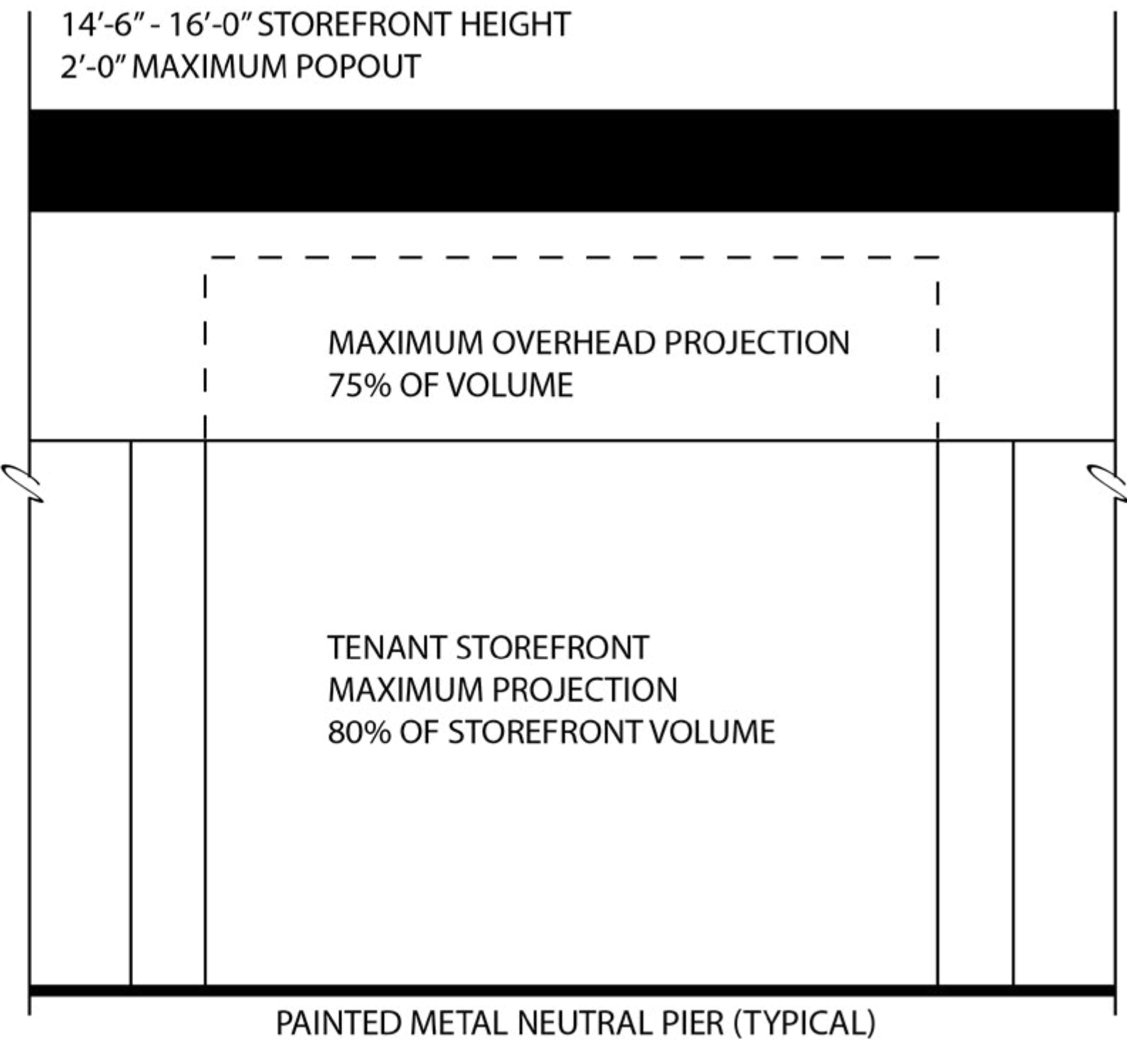
ELEVATION
