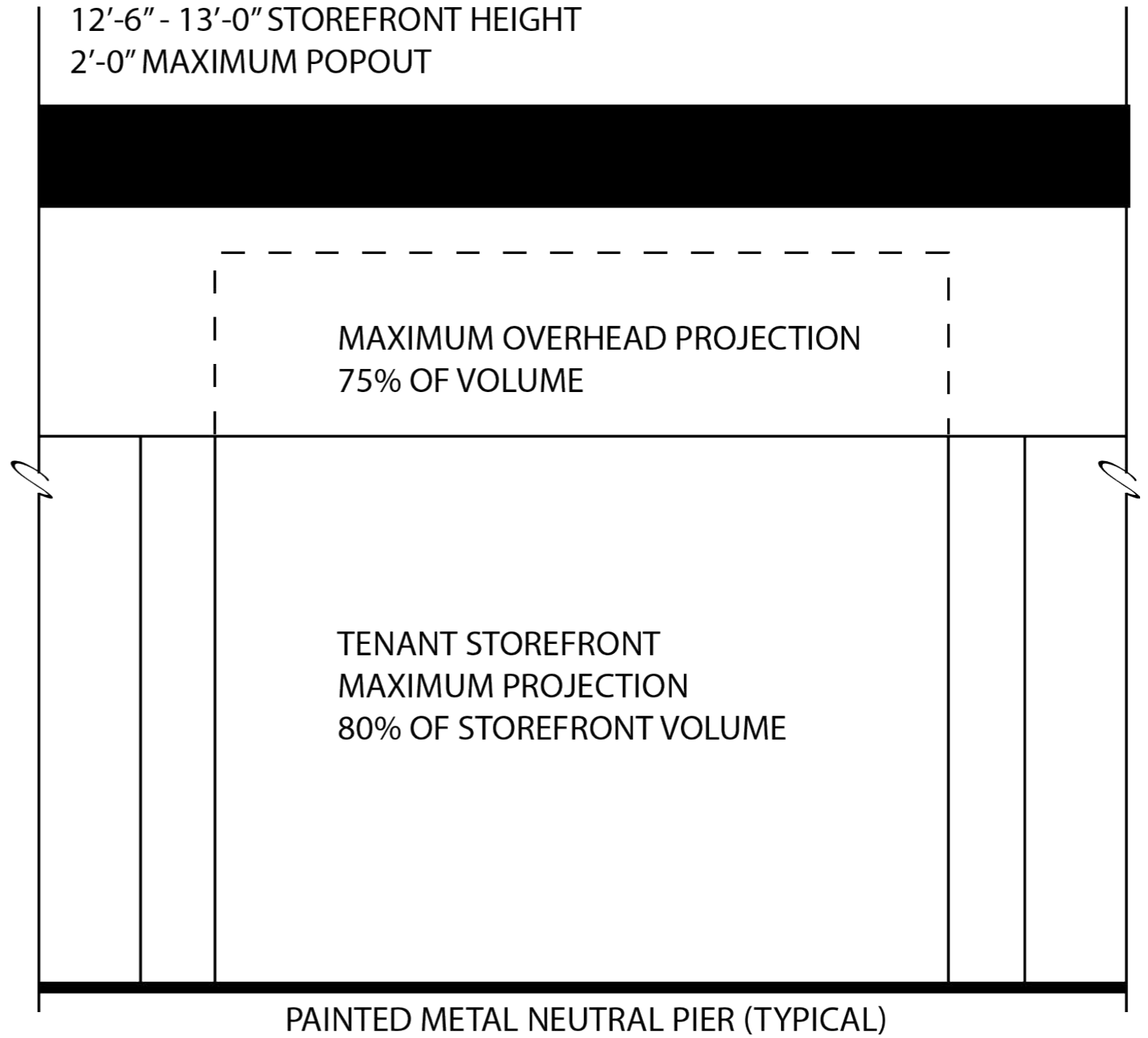
ELEVATION
