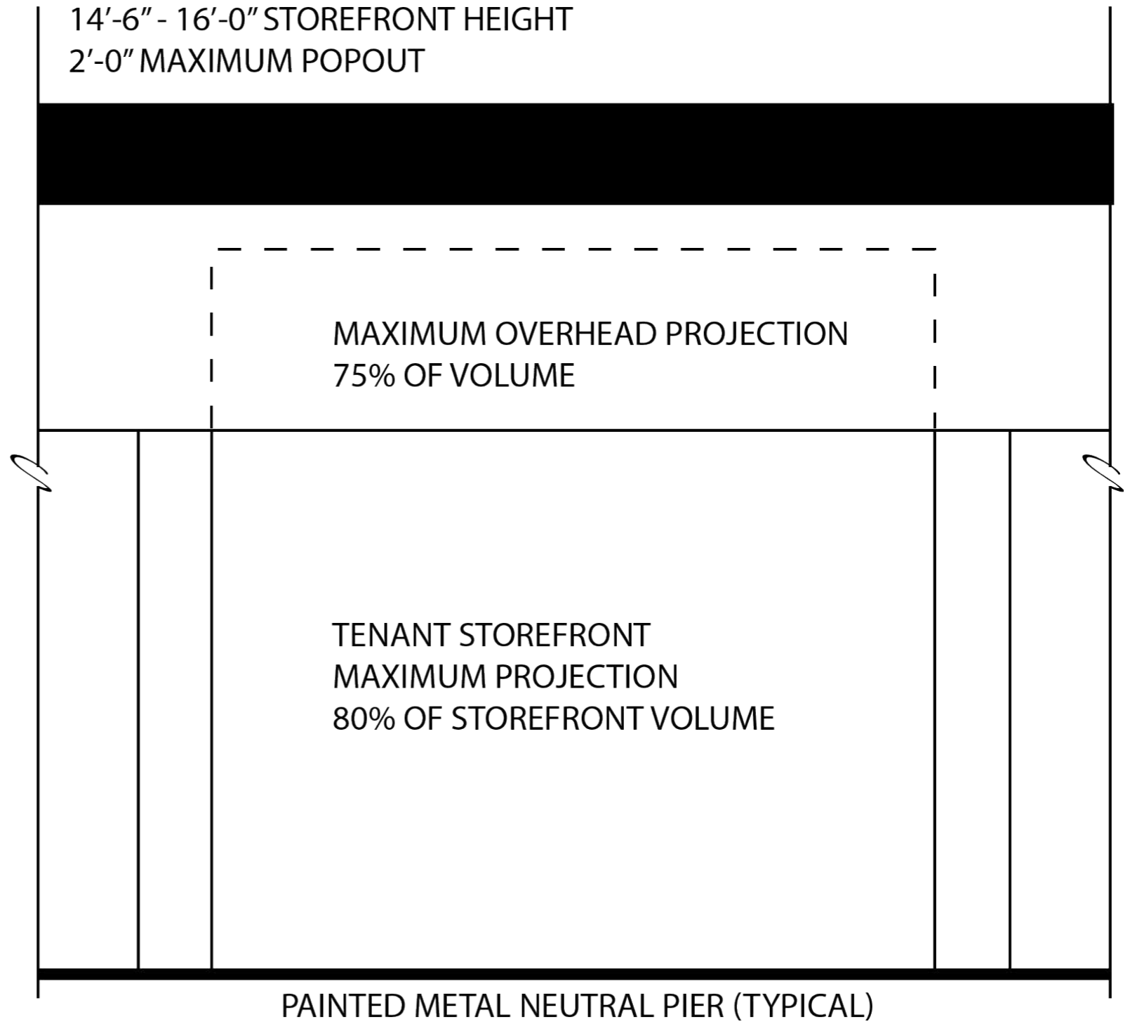
ELEVATION
