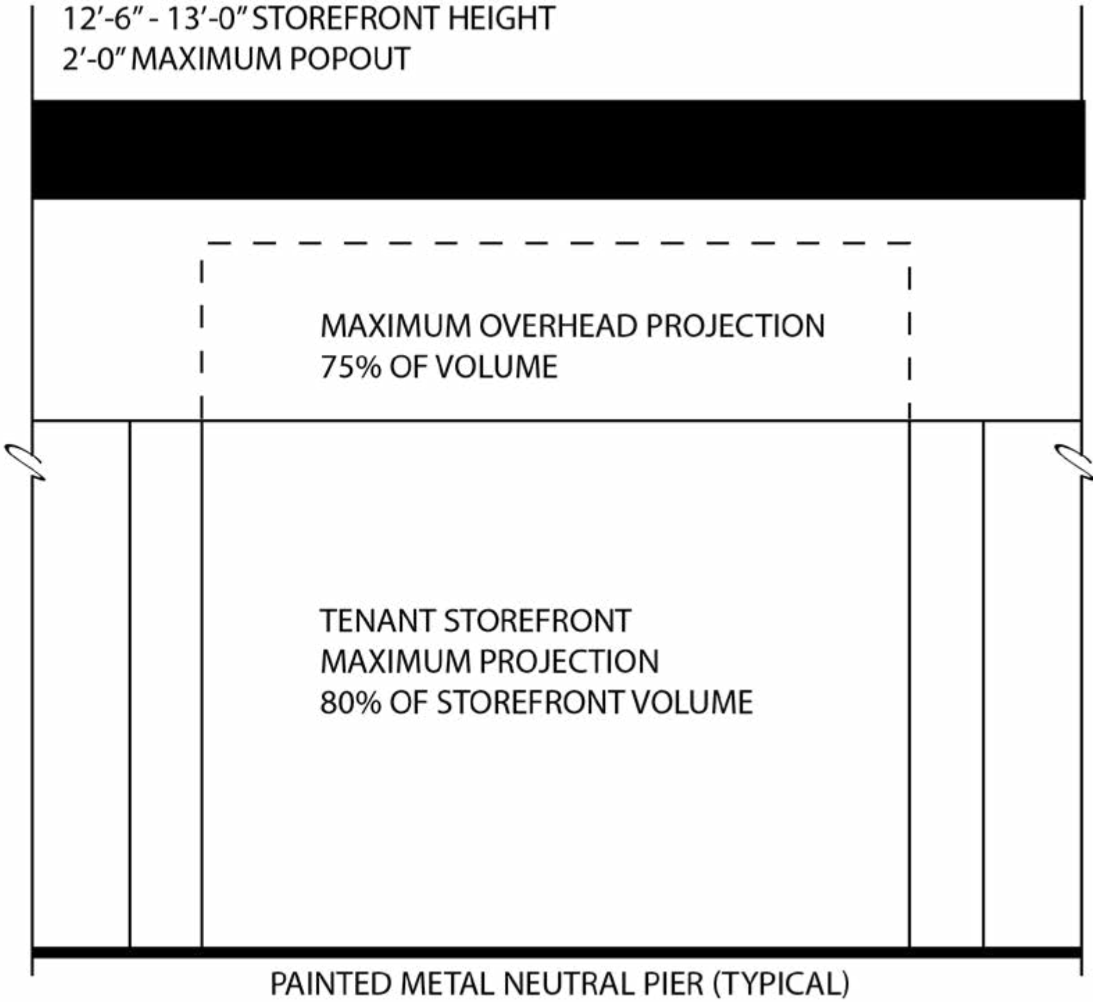
ELEVATION
