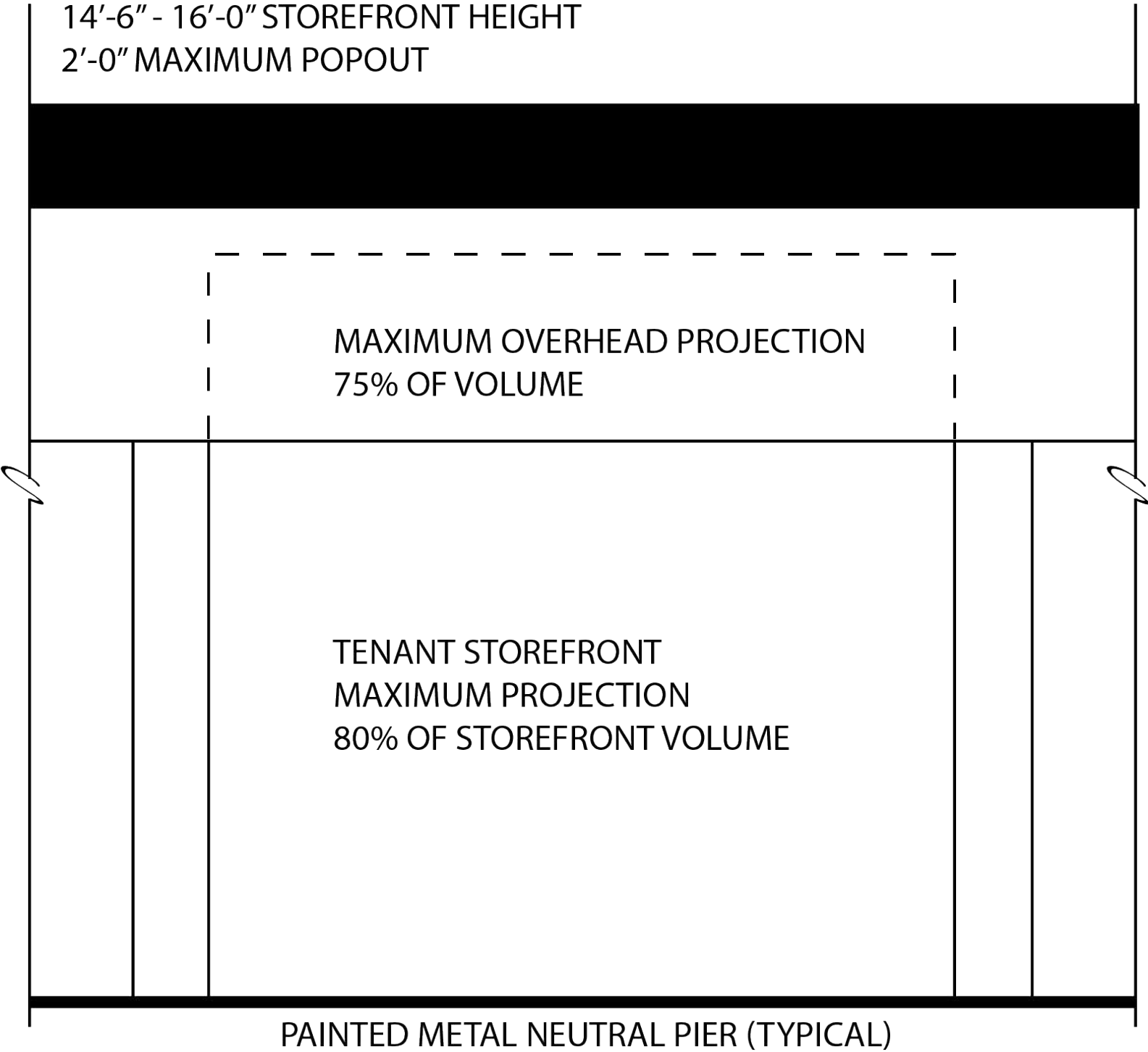
ELEVATION
