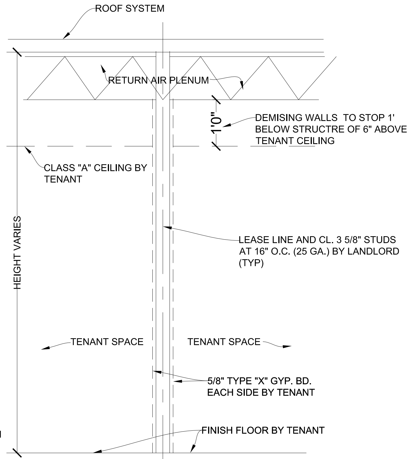
TYP. TENANT DEMISING PARTITION
