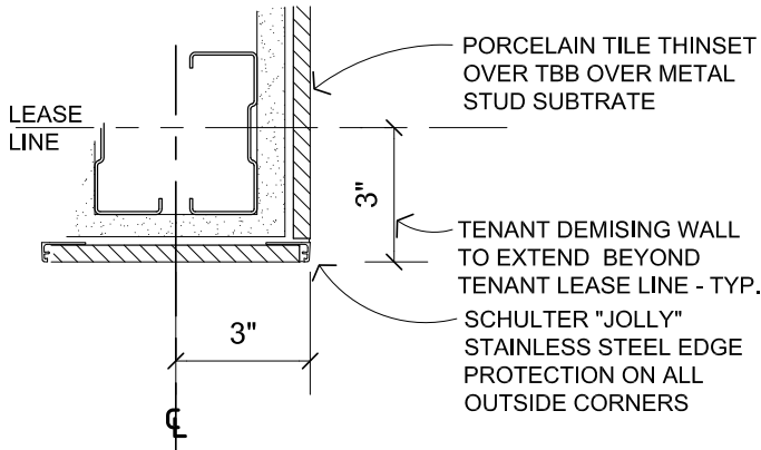
2 CORNER DETAIL SCALE: 3" = 1'-0"
