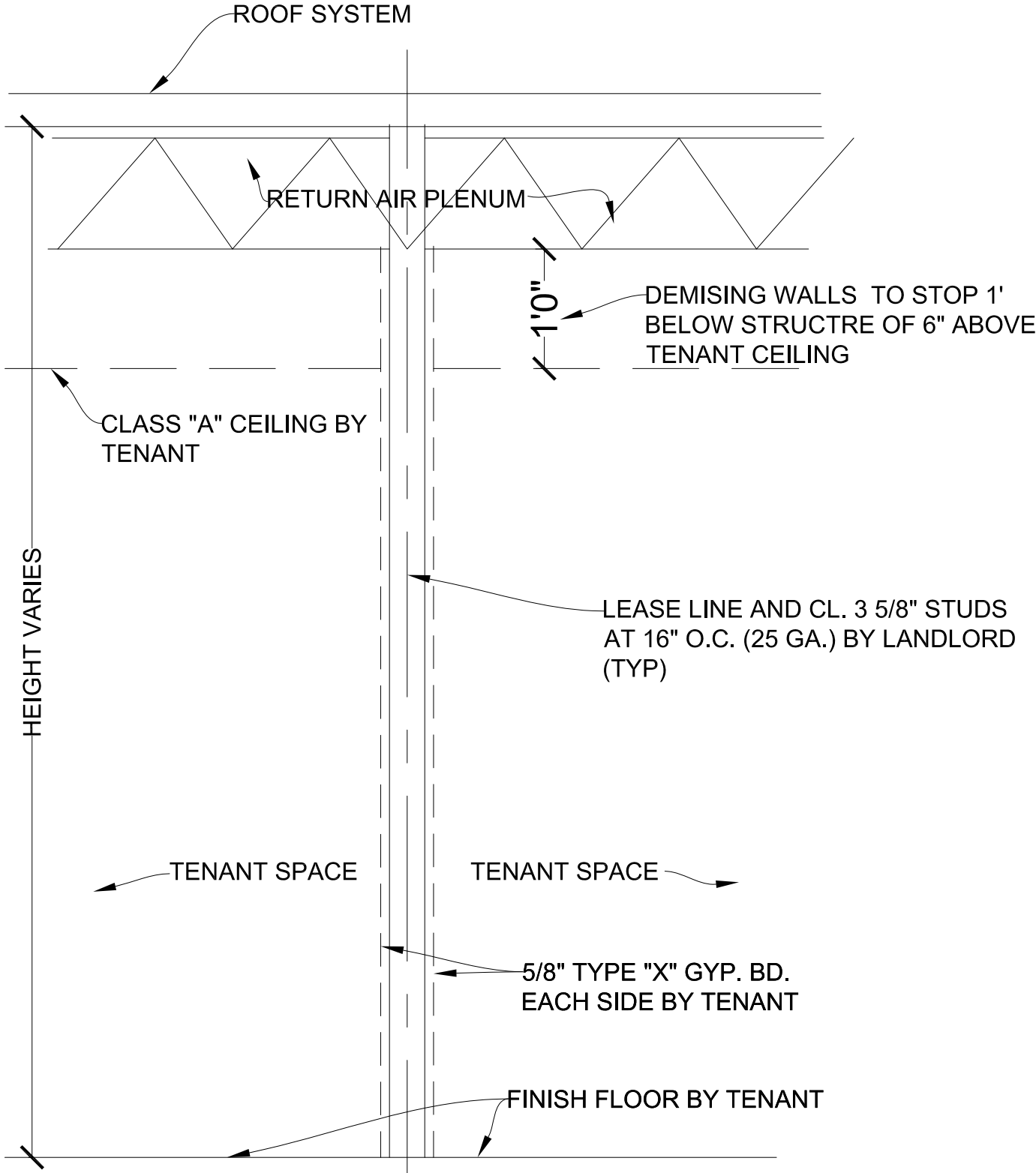
TYP. TENANT DEMISING PARTITION
