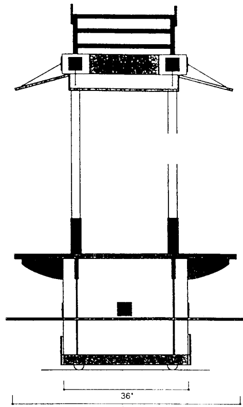
END ELEVATION
