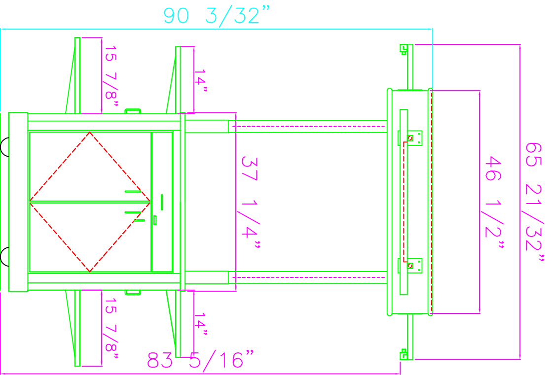
END ELEVATION
