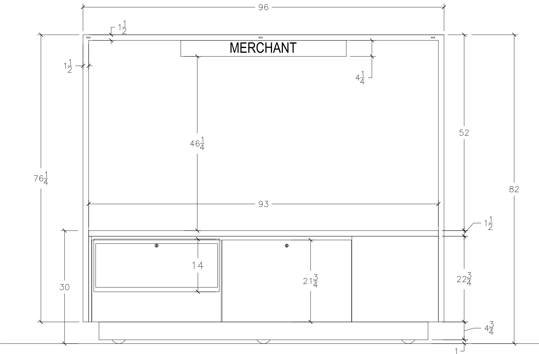
SIDE ELEVATION SCALE: 3/4 " = 1 '
