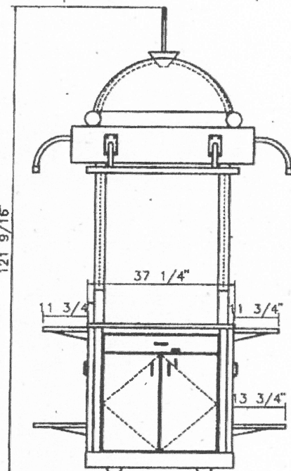
END ELEVATION
