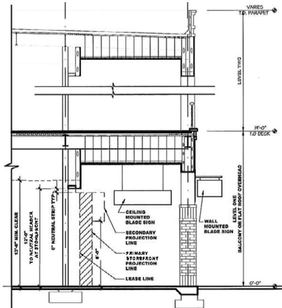
TENANT STOREFRONT ZONES - ZONE 1 - LEVEL ONE SECTION
