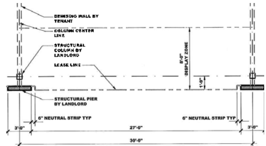
TENANT STOREFRONT ZONES - ZONE 7 - LEVEL TWO PLAN
