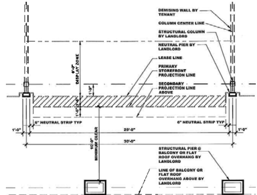
TENANT STOREFRONT ZONES - ZONE 1 - LEVEL ONE PLAN
