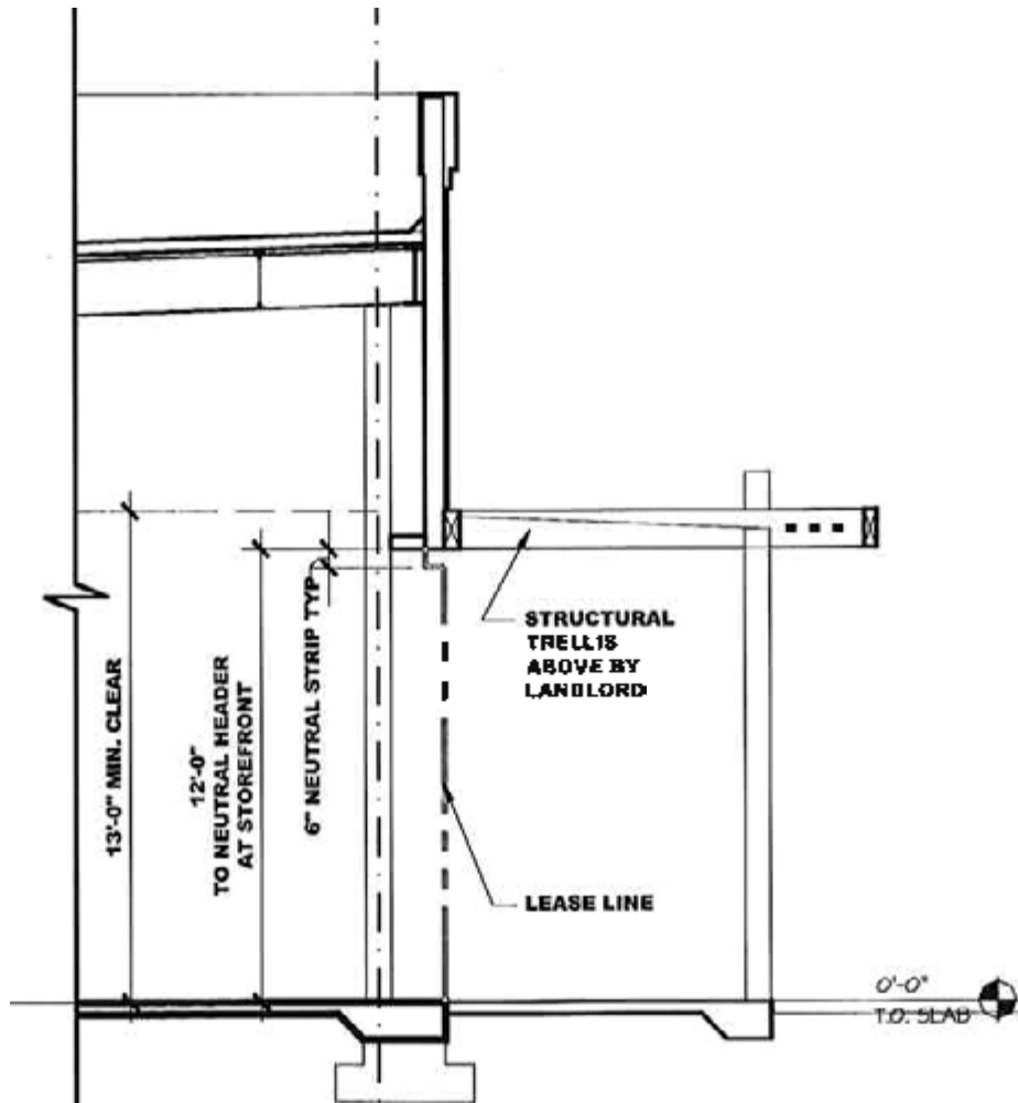
TENANT STOREFRONT ZONES - ZONE 7 - LEVEL TWO SECTION
