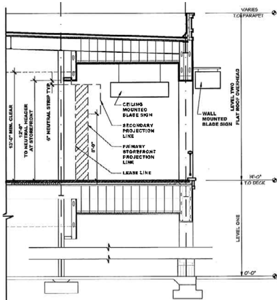
TENANT STOREFRONT ZONES - ZONE 6 - LEVEL TWO SECTION
