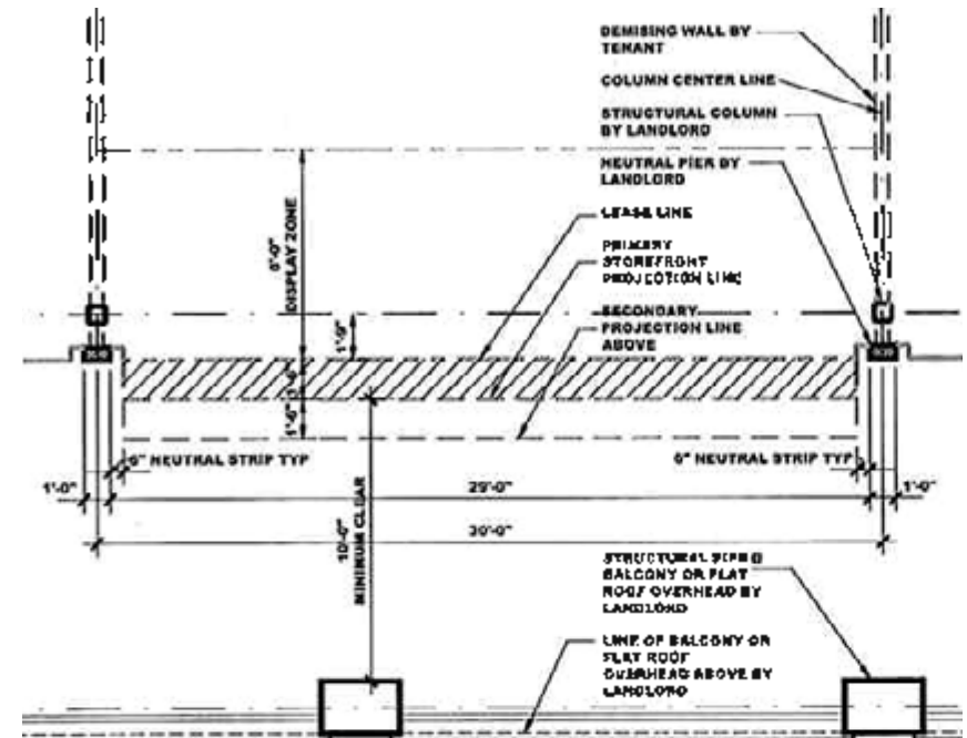
TENANT STOREFRONT ZONES - ZONE 6 - LEVEL TWO PLAN
