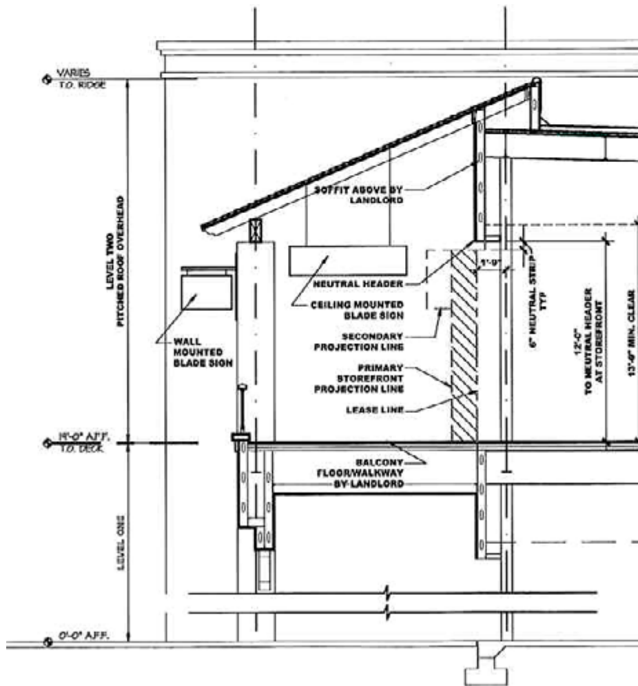
TENANT STOREFRONT ZONES - ZONE 5 - LEVEL TWO SECTION
