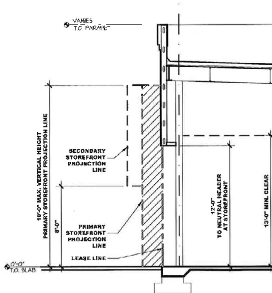
TENANT STOREFRONT ZONES - ZONE 4 - LEVEL TWO SECTION
