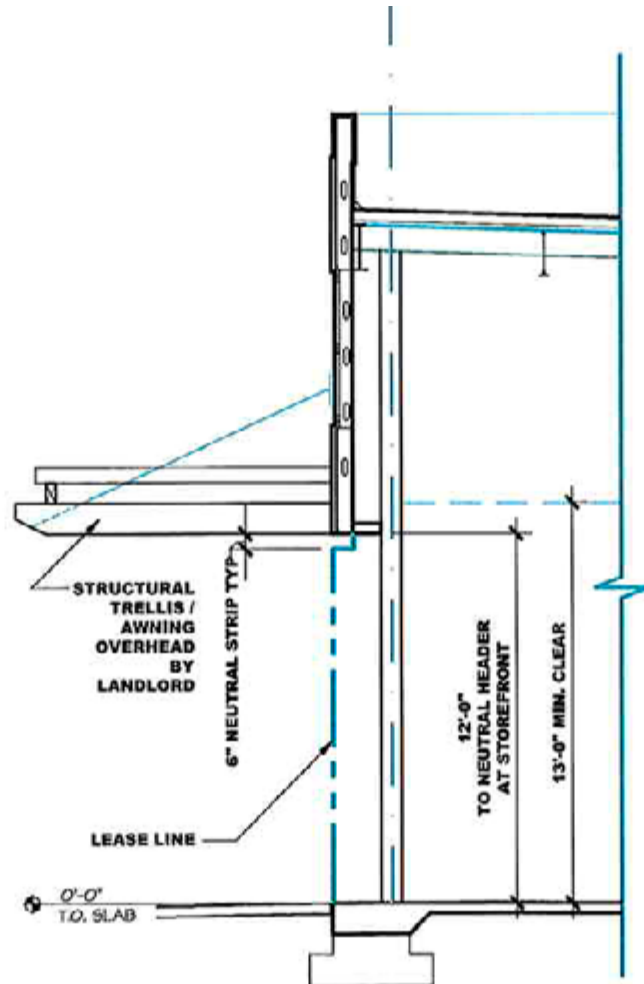
TENANT STOREFRONT ZONES - ZONE 2 - LEVEL ONE SECTION
