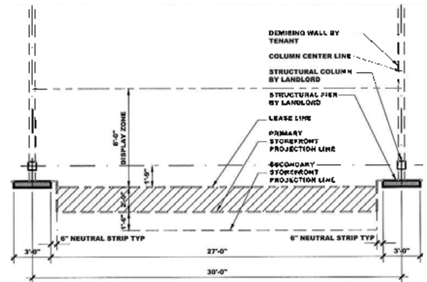
TENANT STOREFRONT ZONES - ZONE 4 - LEVEL TWO PLAN
