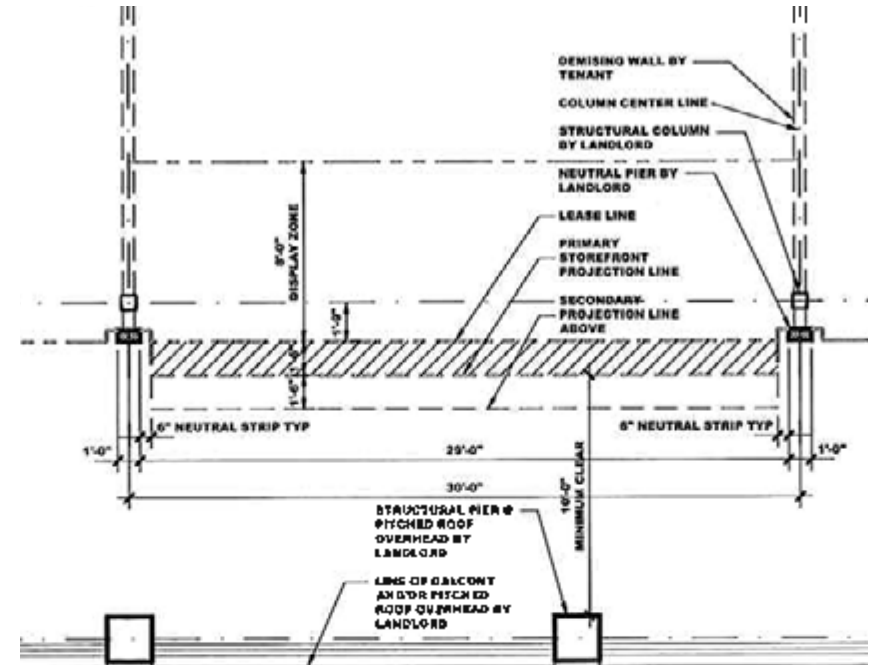
TENANT STOREFRONT ZONES - ZONE 5 - LEVEL TWO PLAN
