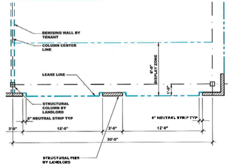
TENANT STOREFRONT ZONES - ZONE 2 - LEVEL ONE PLAN
