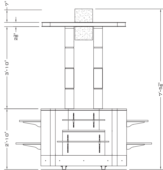
ELEV 4 END ELEVATION SCALE: 3/4"=1'-0"
